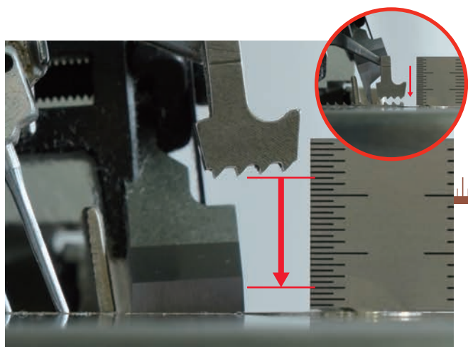
·上送布的上下运动量为 9.5 毫米
