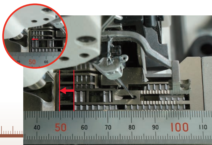
·最大缝距 6mm
